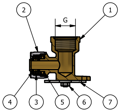
A-A ( 1 : 2 )
